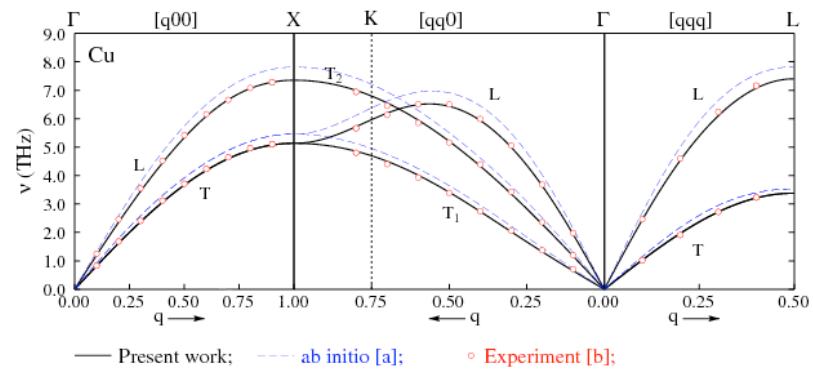
fcc Cu
